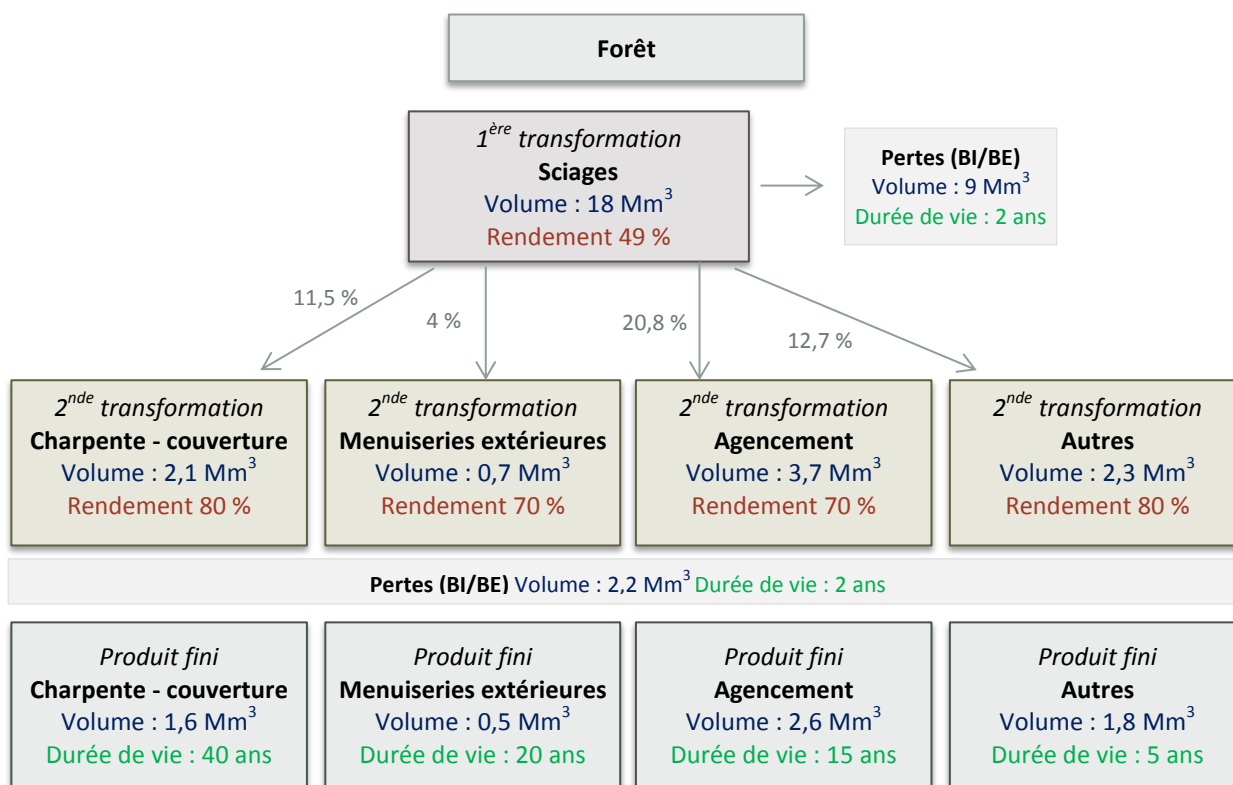
Figure 17. Analyse du cycle de vie d'un produit de construction bois (d'après Vallet, 2005)
