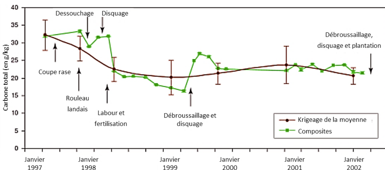
Figure 14. Évolution des teneurs en carbone organique total dans le sol après une coupe rase (Landes) (Jolivet, 2000 in Citeau & al. , 2008)
