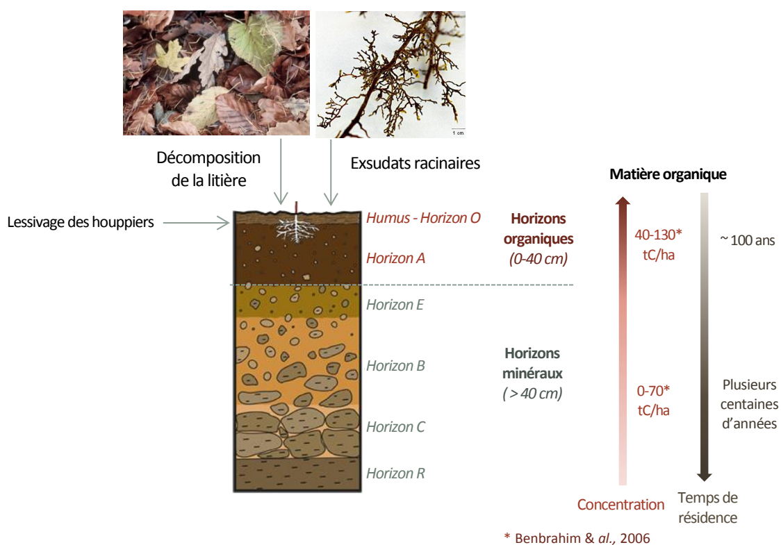
Figure 3. Concentration en carbone et temps de résidence de la matière organique dans un sol forestier
