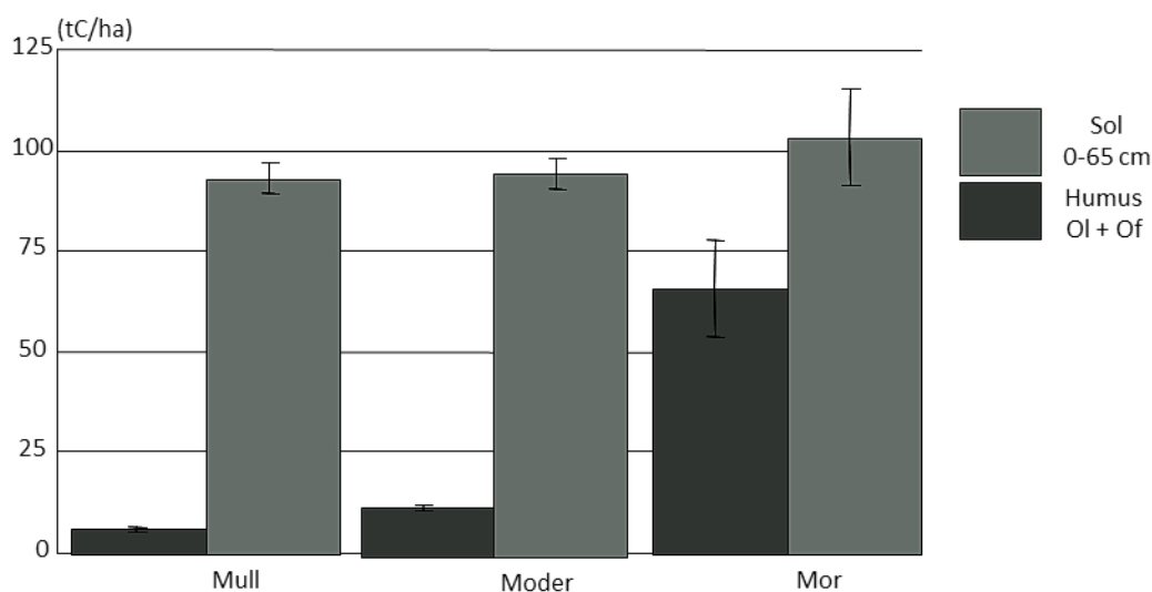
Figure 2. Répartition du carbone pour les 3 types d'humus ( Nys & al., 2002)
