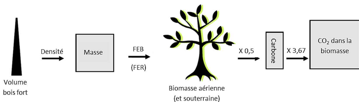
Figure 4. Calcul de la quantité de carbone dans la biomasse
