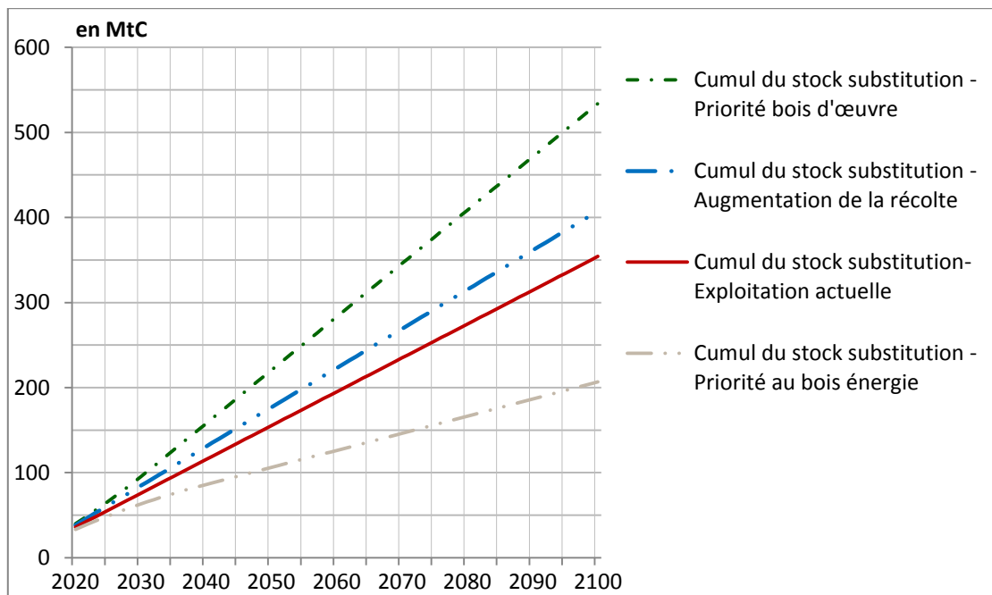
Figure 2. Modélisation de l'évolution du cumul des économies de carbone dues à l'utilisation de bois d'œuvre et de bois d'industrie récoltés en France en substitution à d'autres matériaux
