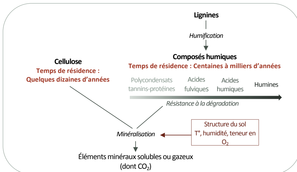
Figure 1. Évolution de la matière organique du sol
