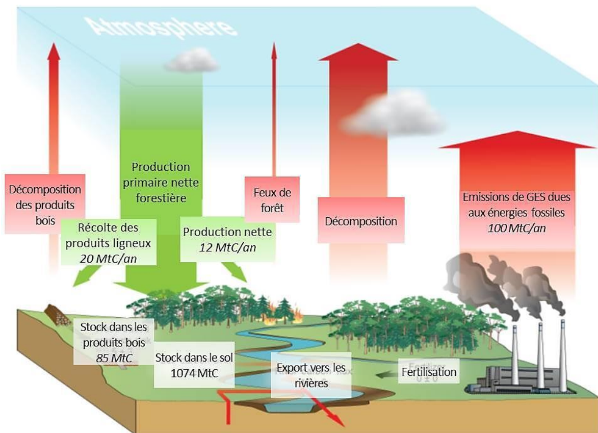
Figure 5. Les flux de carbone forestier pour la France en regard des émissions de GES dues aux énergies fossiles (d'après Luyssaert & al., 2010)
