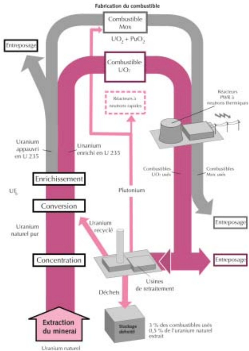
Cycle simplifié du combustible nucléaire en France
